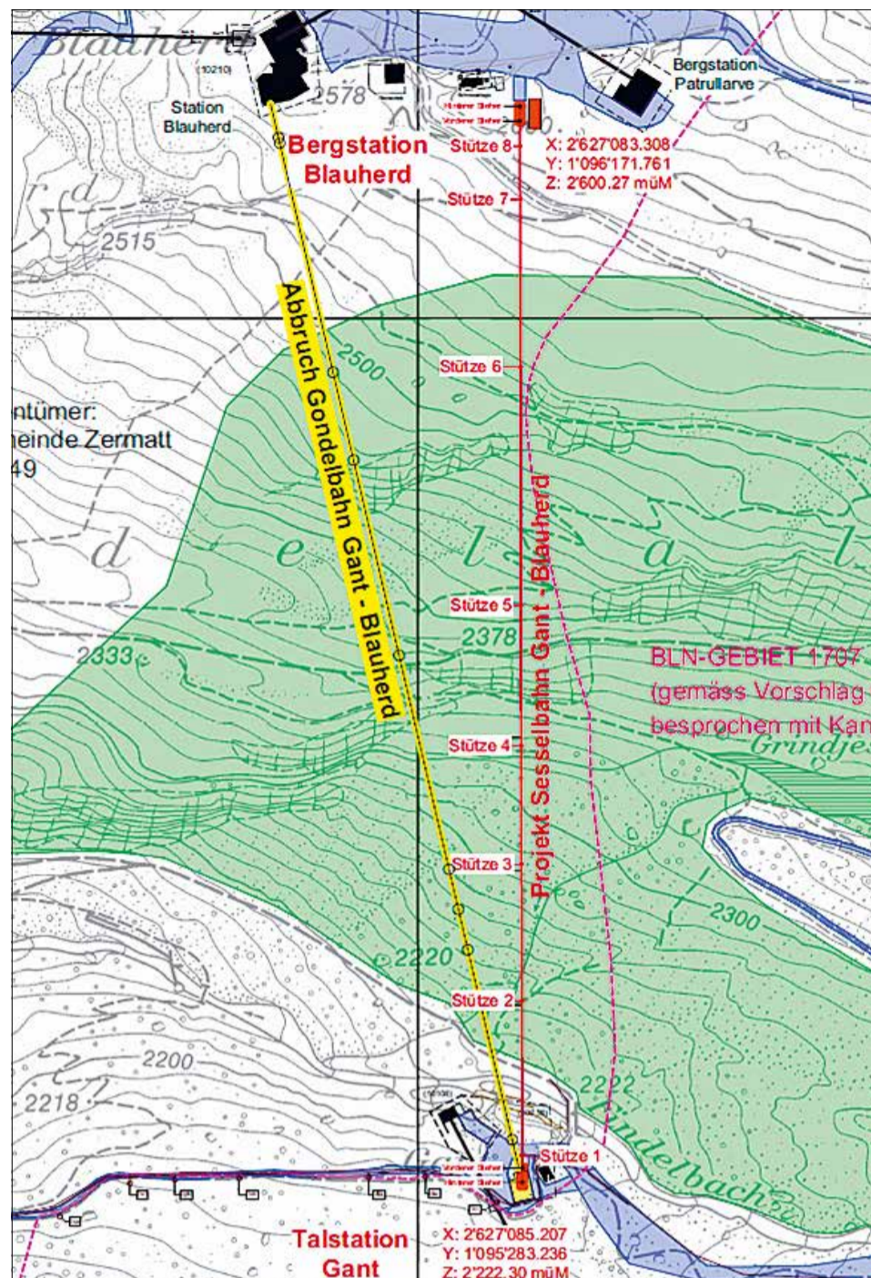
Standortskizze der alten und der neuen Anlage.
