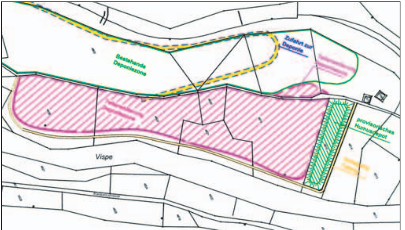
Die dringend nötige Deponie-Erweiterung II Zum Biel umfasst eine Fläche von 18 000 m 2 und ein Volumen von 170 000 m 3 .
